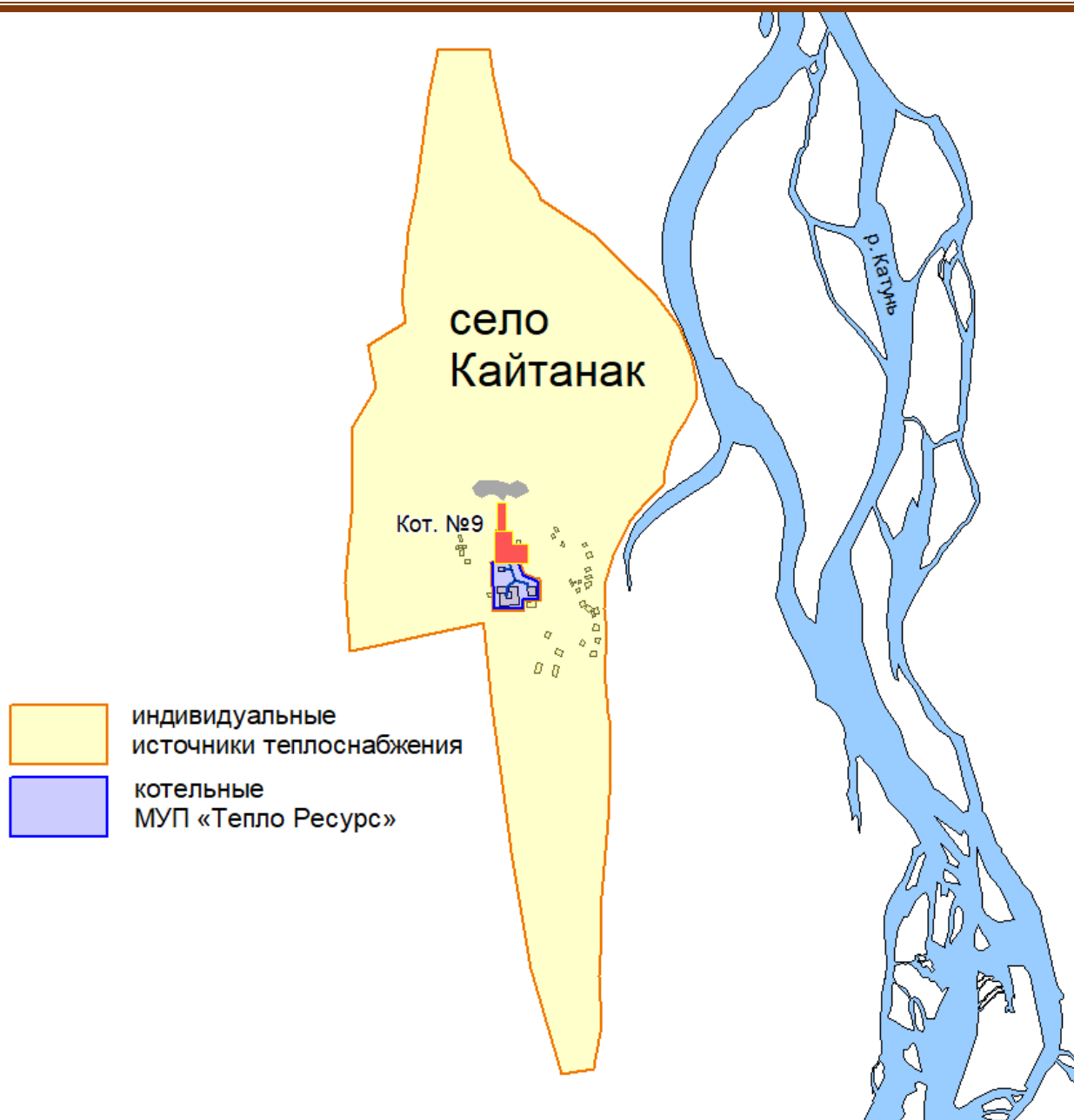
Рисунок 2.8 – Зона действия источников тепловой энергии с. Кайтанак
