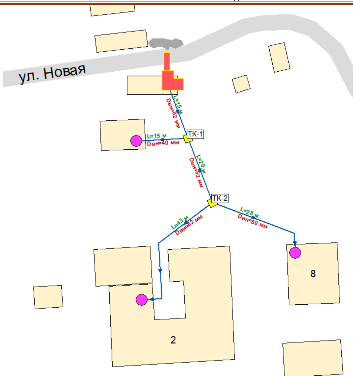
Рисунок 2.6 – Схема тепловых сетей в зоне действия котельной №9, с. Кайтанак
