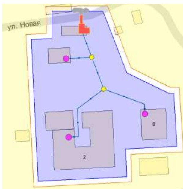
Рисунок 4.7 – Зона действия котельной №9 (с. Кайтанак)
