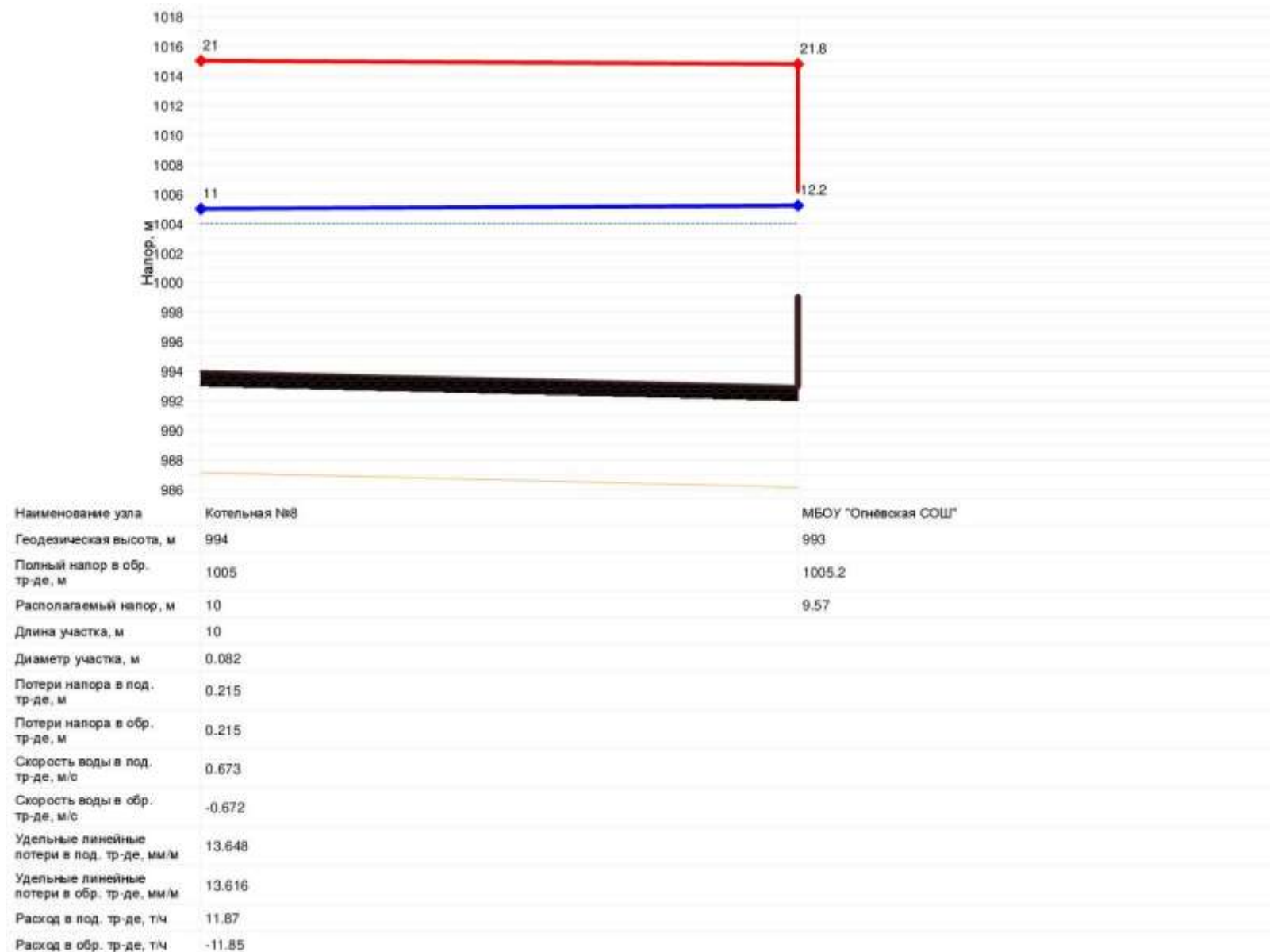
Рисунок 4.18 – Пьезометрический график от котельной №8 до школы (ул. Школьная, 8, с. Огнёвка)
