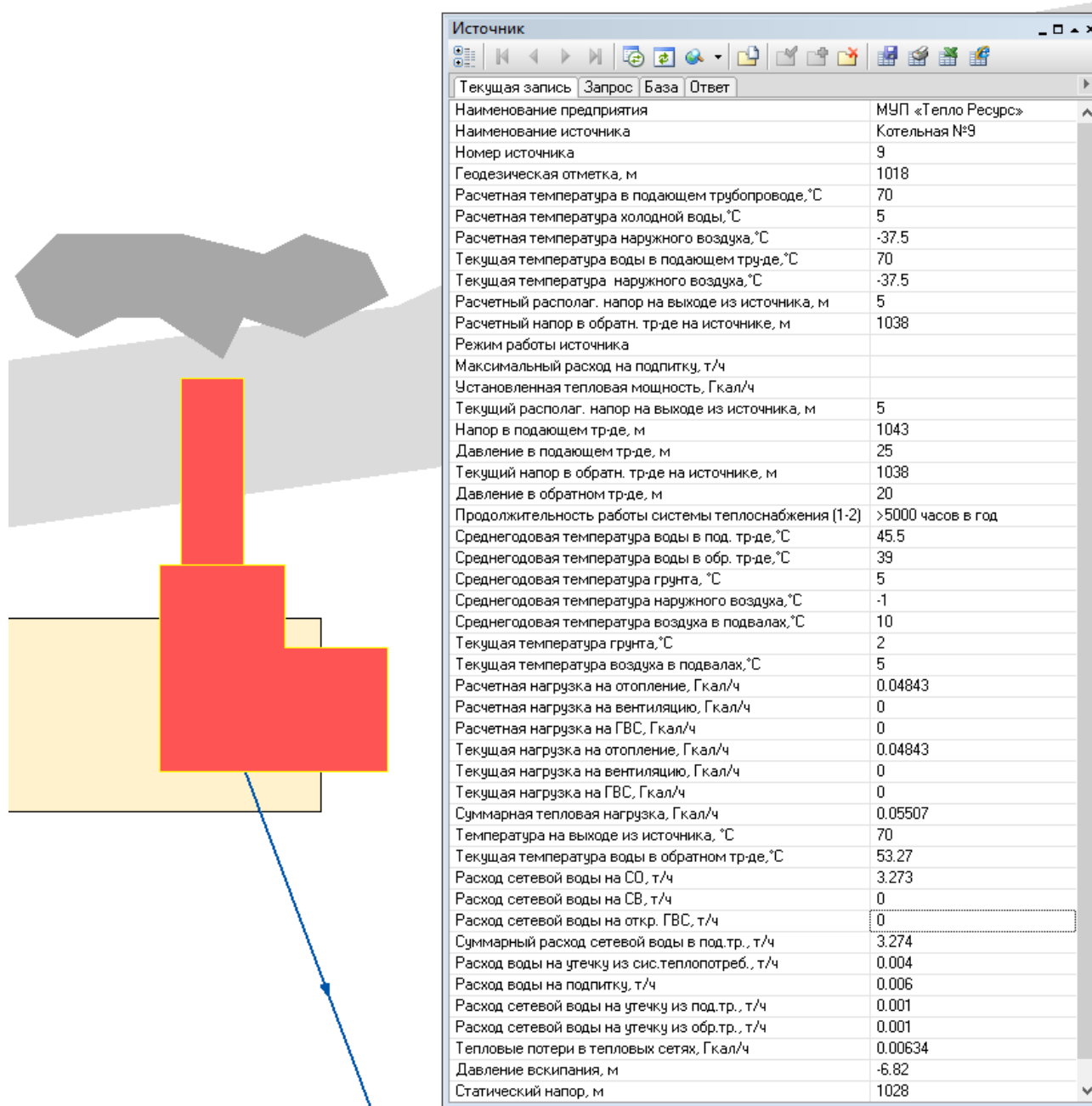
Рисунок 4.4 – Пример отображения источника тепловой энергии
