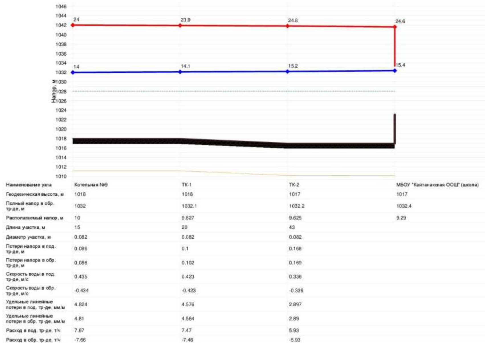
Рисунок 4.19 – Пьезометрический график от котельной №9 до школы (ул. Новая, 2, с. Кайтанак)
